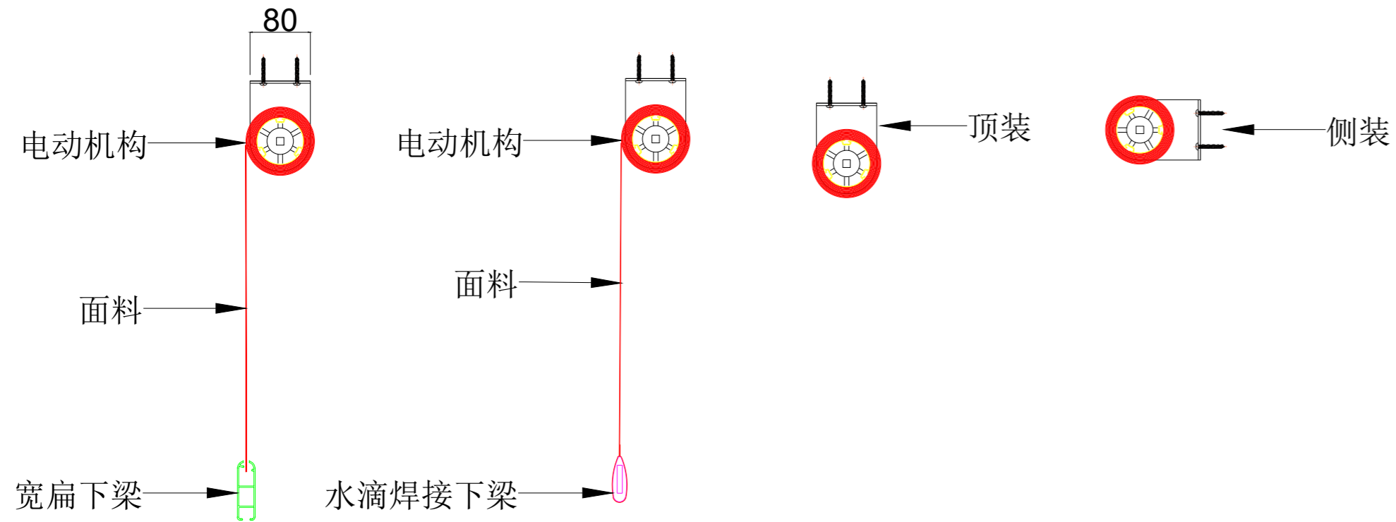
电动卷帘产品安装剖面图
